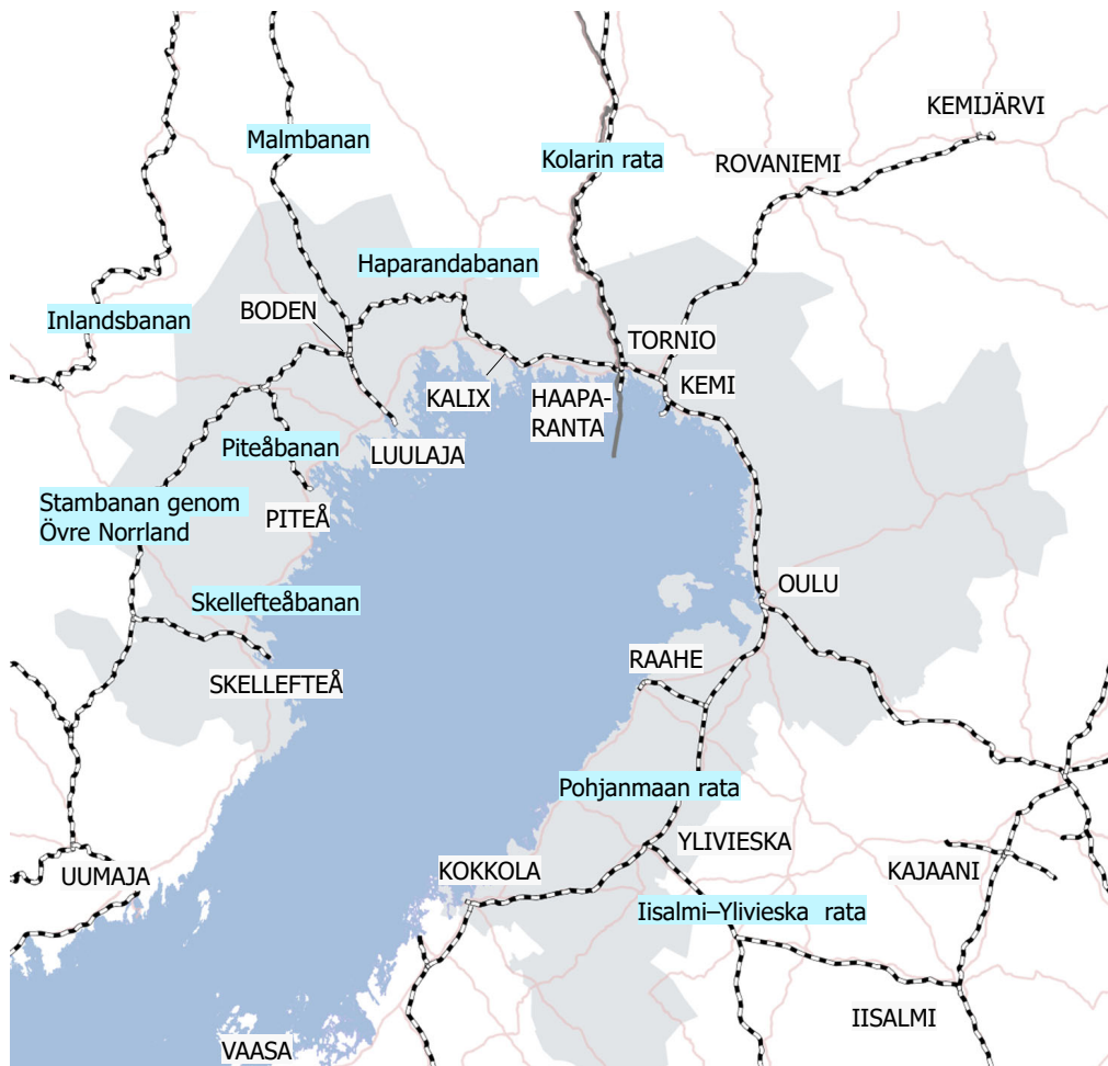
Kuva 4. Perämerenkaaren rataverkko.
